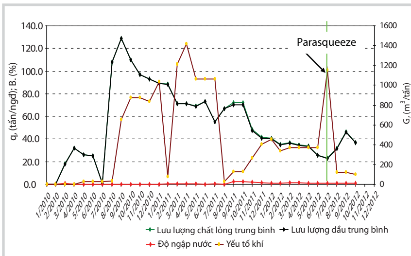
Hình 2. Động thái làm việc của giếng R81 trước và sau khi áp dụng công nghệ "Parasqueeze"
