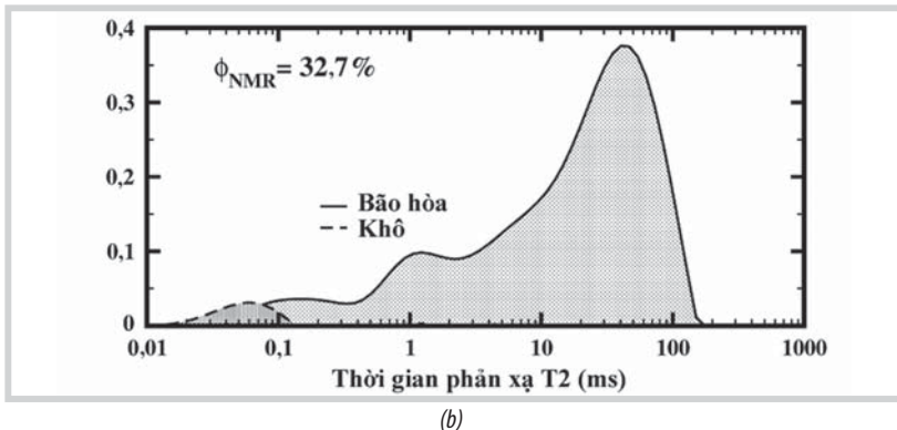
Hình 4. Phân bố bán kính hạt trong mẫu OSS bằng đo nhiễu xạ ánh sáng, đa số các hạt có bán kính 58μm, phân bố bán kính lỗ rỗng, đa số có bán kính 9μm và nhỏ nhất là 0,01 μm (a); phân bố thời gian hồi phục T2 bằng kỹ thuật NMR cho mẫu OSS khô và mẫu bão hòa (b).
