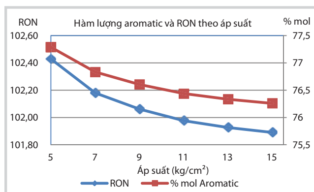
Hình 13. Sự thay đổi chất lượng reformate khi áp suất thay đổi
