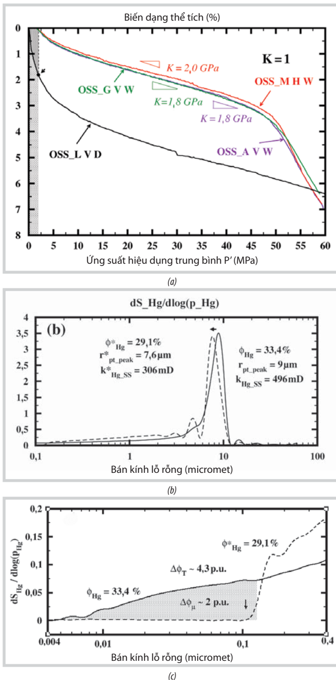
Hình 8. Thí nghiệm nén đẳng hướng trên mẫu khô thẳng đứng, mẫu thẳng đứng và ngang bão hòa bằng nước muối NaCl (a); Phân bố kích thước lỗ rỗng trên mẫu OSS_A V W (điểm cực đại tại bán kính 7,6 \mu m) được so sánh với mẫu nguyên dạng trong Hình 4a (b); Sự giảm các lỗ rỗng sau khi nén (c)
